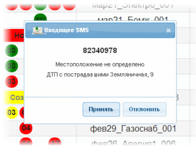
Рисунок 5-7: Приём SMS-обращения
