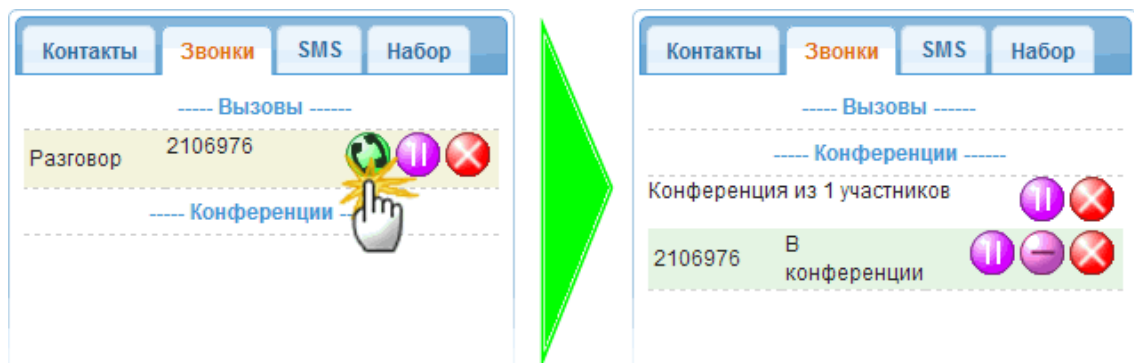
Рисунок 5-23: Создание конференции
